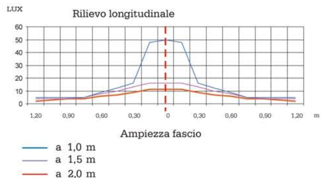
Curve fotometriche
