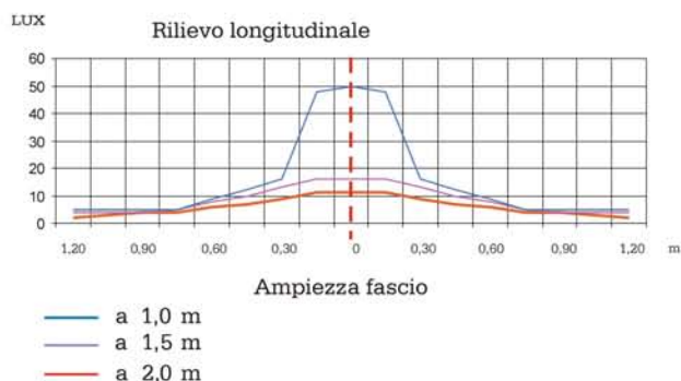
Curve fotometriche
