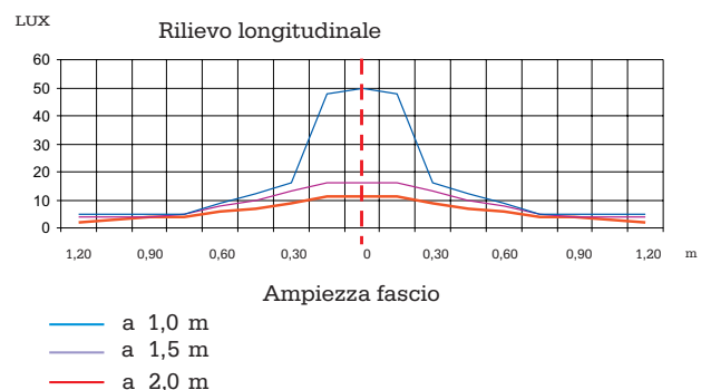
Curve fotometriche
